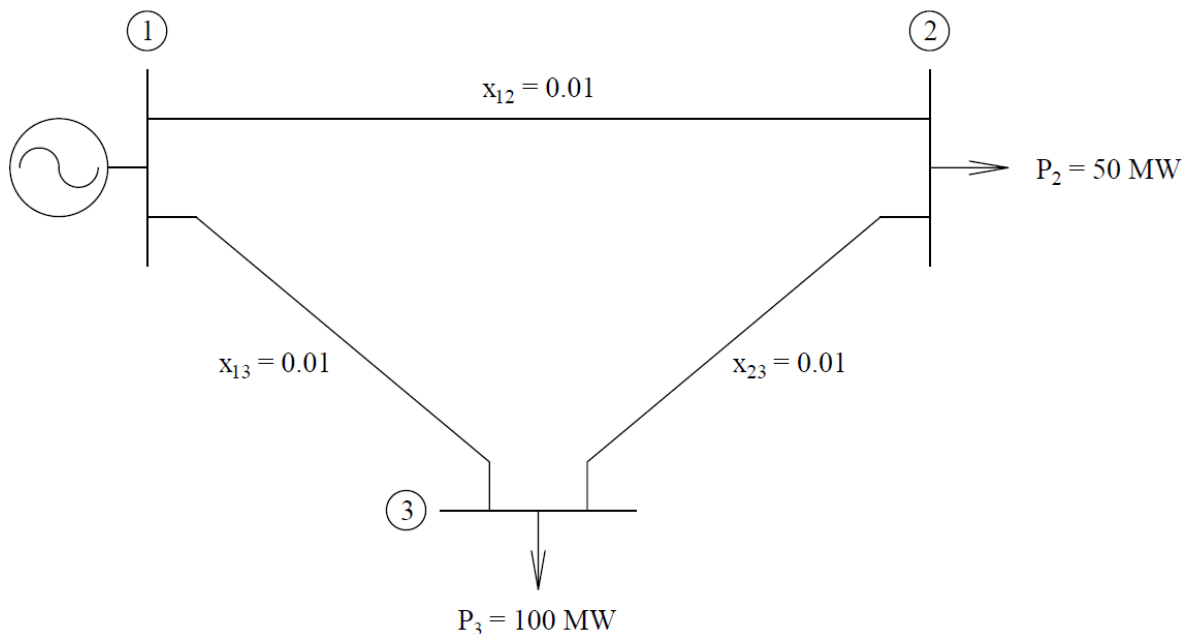
Slika 1. Jednopolna šema elektroenergetskog sistema
